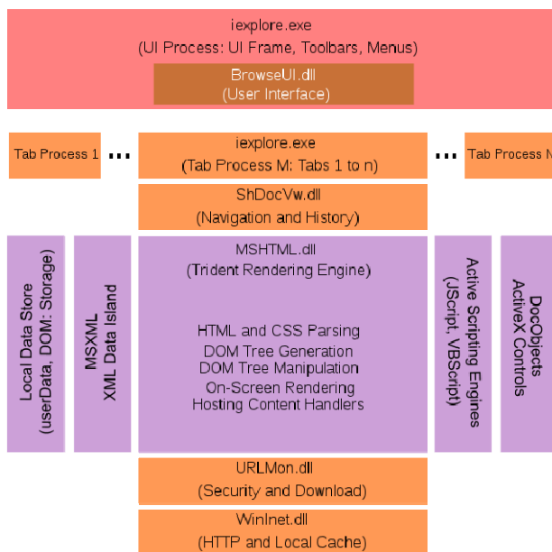
IE 8 的架构
