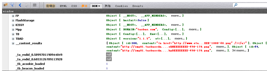
Firebug 的界面
