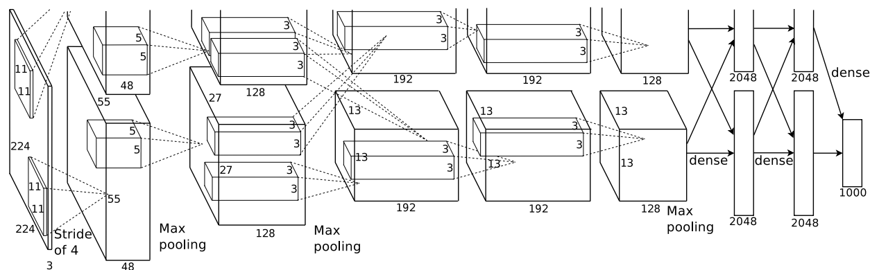
图10.5.1: 由于GPU显存有限，原有AlexNet设计中的模型并行。
