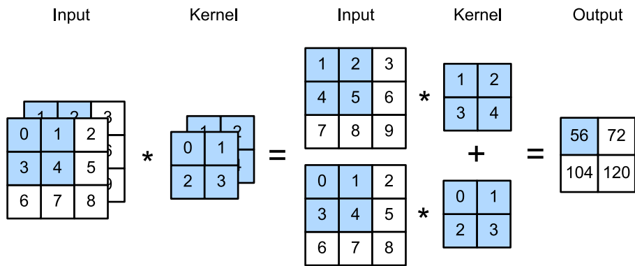
图6.4.1: 两个输入通道的互相关计算。
