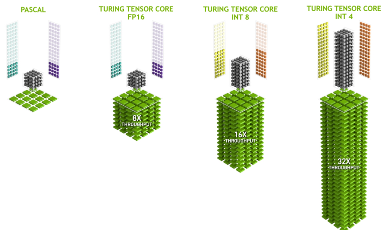
图10.4.9: NVIDIA Turing架构中的张量核心（图片由英伟达提供）
