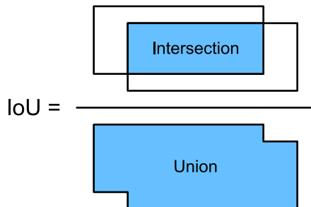
图11.4.1: 交并比是两个边界框相交面积与相并面积之比。
