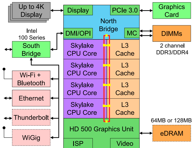
图10.4.3: Intel Skylake消费级四核CPU。
