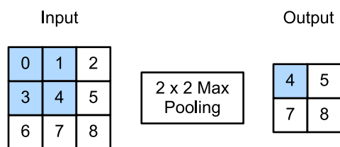
图6.5.1: 池化窗口形状为 2 \times 2 的最大池化层。着色部分是第一个输出元素，以及用于计算这个输出的输入元素: \max(0, 1, 3, 4) = 4 .
