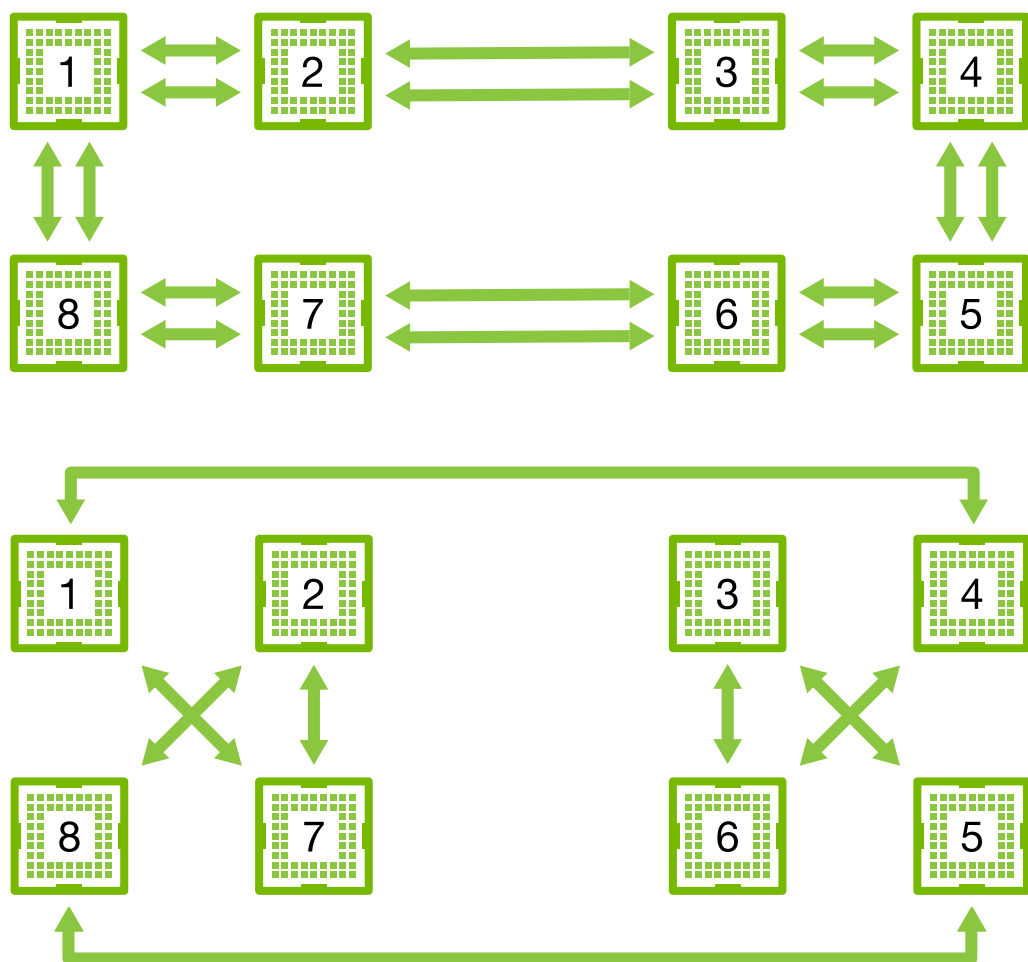
图10.7.5: 将 NVLink 网络分解为两个环。
