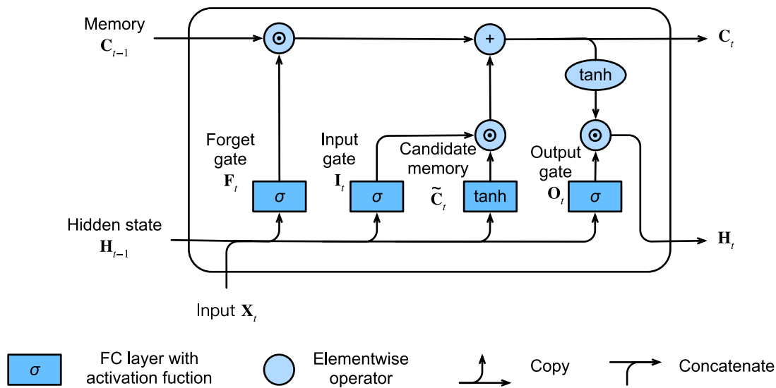
图9.2.4: 在长短期记忆模型中计算隐藏状态。
