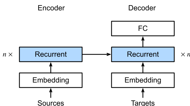
图9.7.2: 循环神经网络编码器-解码器模型中的层。
