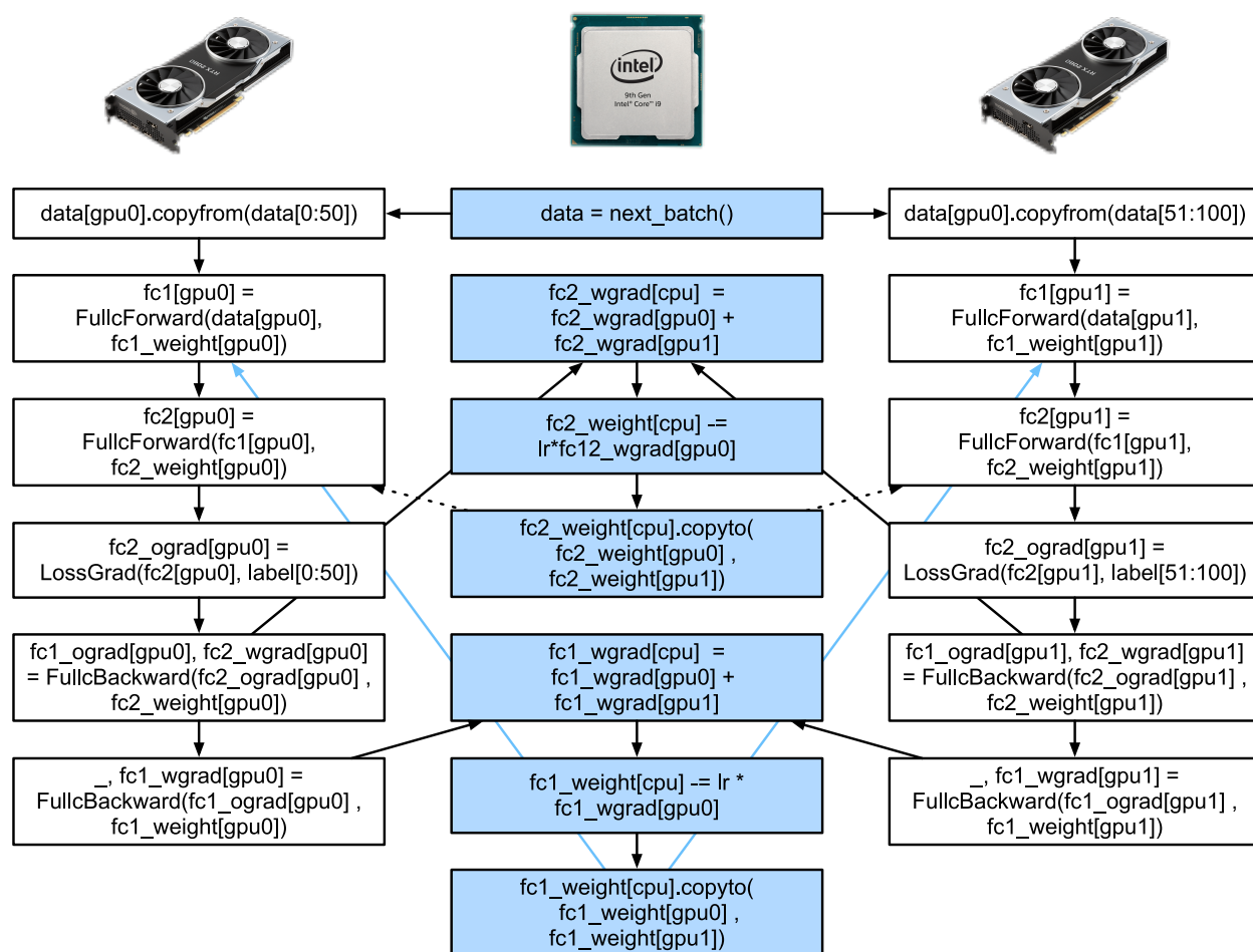
图10.3.1: 在一个 CPU 和两个 GPU 上的两层的多层感知机的计算图及其依赖关系。
