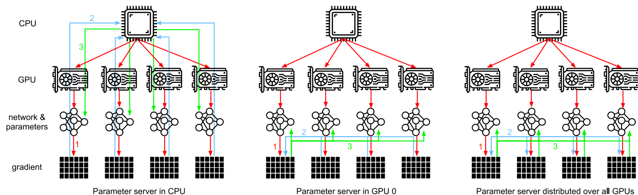
图10.7.3: 参数同步策略
