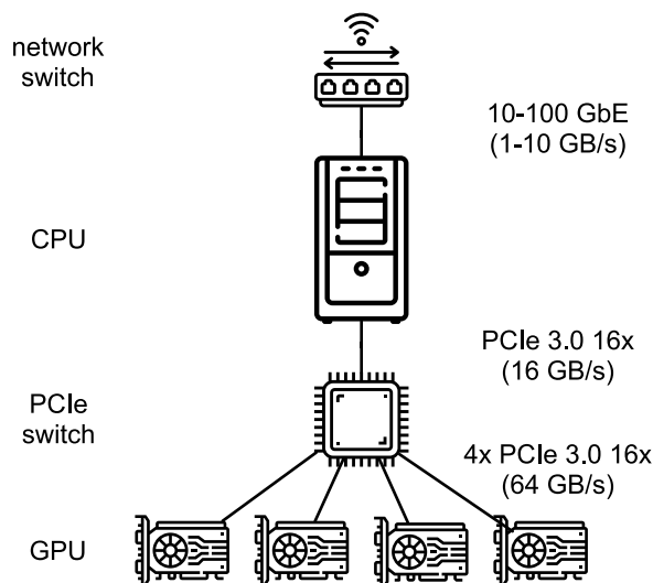
图10.7.2: 一个4路GPU服务器
