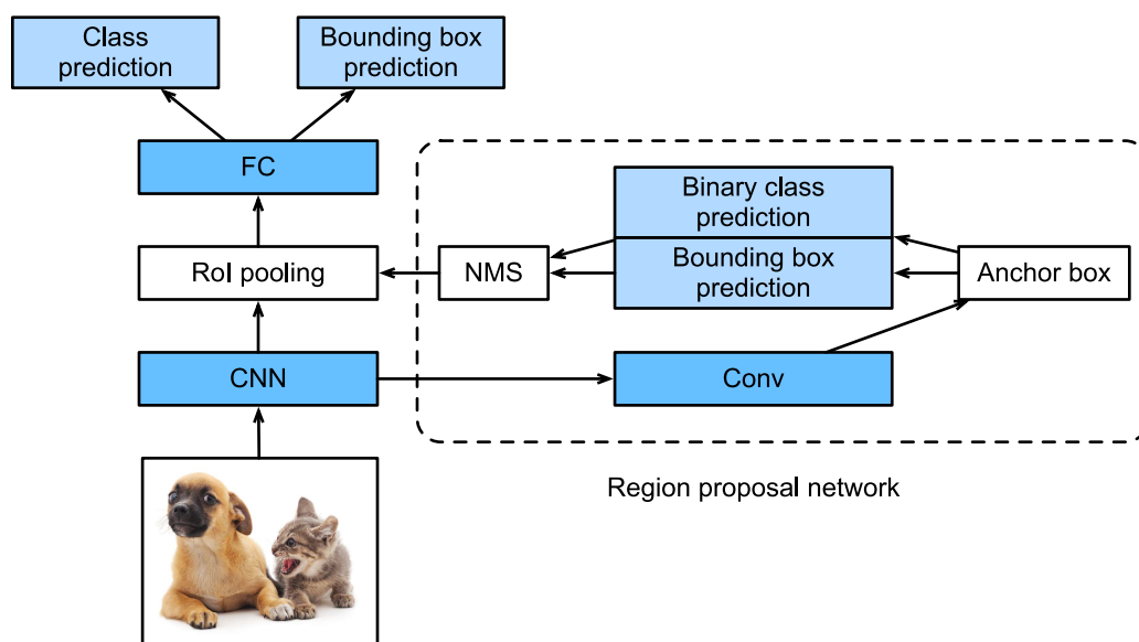
图11.8.4: Faster R-CNN 模型
