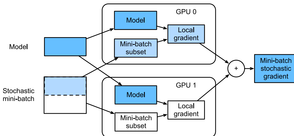
图10.5.3: 利用两个GPU上的数据，并行计算小批量随机梯度下降。
