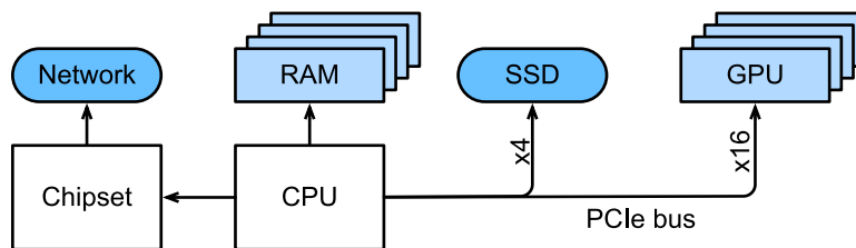
图10.4.2: 计算机组件的连接。
