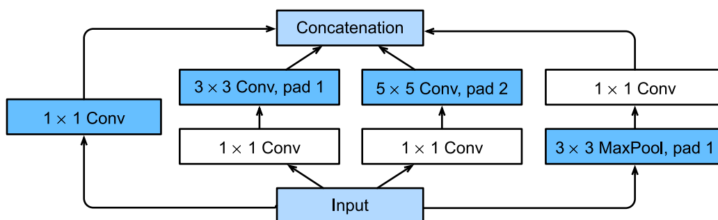
图7.4.1: Inception块的结构。
