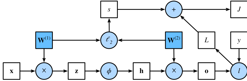
图4.7.1: 正向传播的计算图
