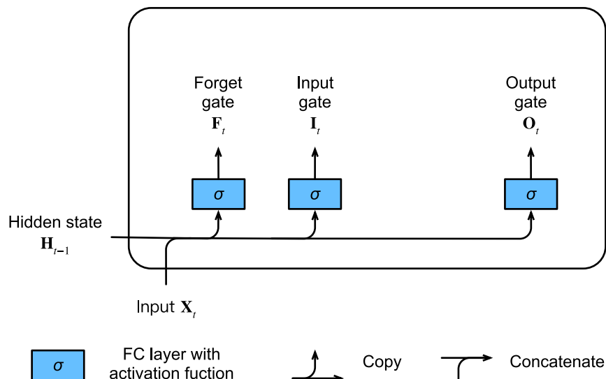
图9.2.1: 在长短期记忆模型中计算输入门、遗忘门和输出门。
