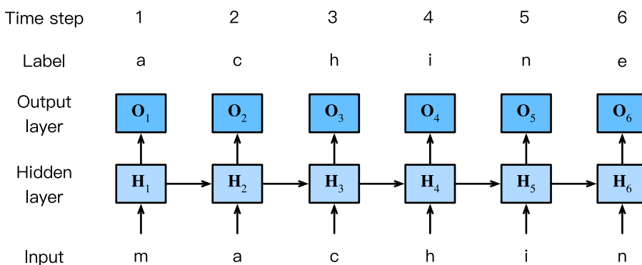
图 8.4.2: 基于循环神经网络的字符级语言模型。输入序列和标签序列分别为 “machin” 和 “achine”。
