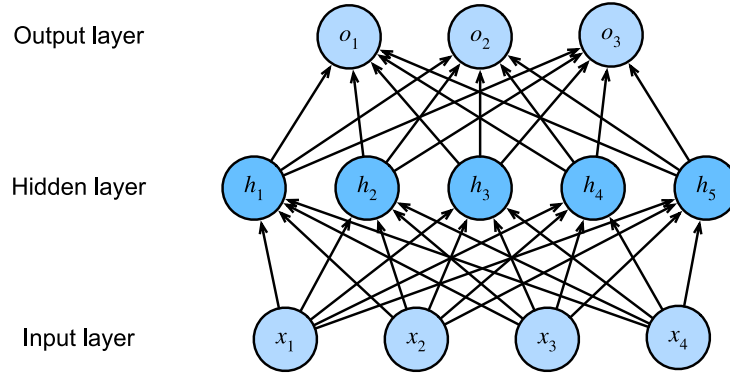
图4.1.1: 一个单隐藏层的多层感知机，具有5个隐藏单元
