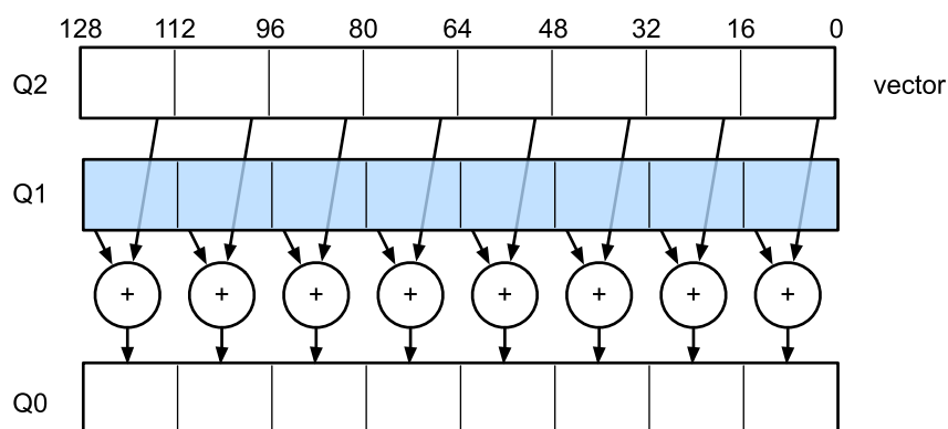
图10.4.5: 128位NEON矢量化
