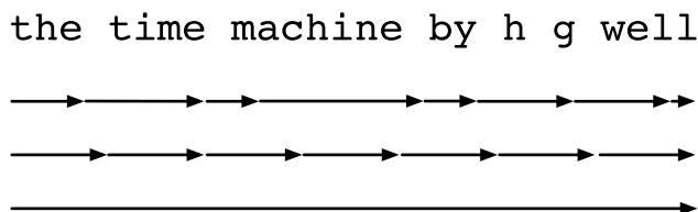
图8.7.1: 比较RNN中计算梯度的策略。自上而下：随机截断、常规截断、完整计算。
