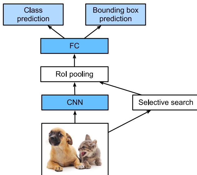
图11.8.2: Fast R-CNN模型
