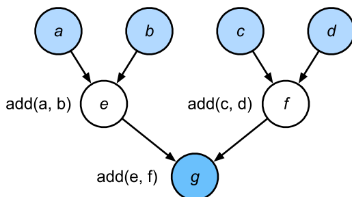
图10.1.1: 命令式编程中的数据流。
