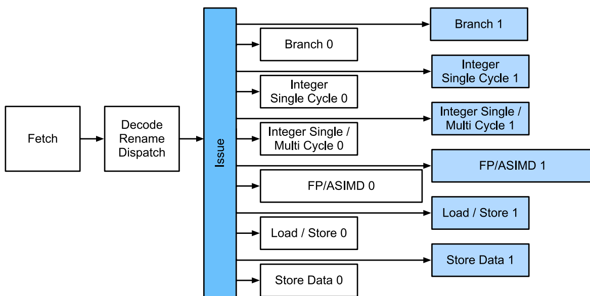
图10.4.4: ARM Cortex A77 微体系结构
