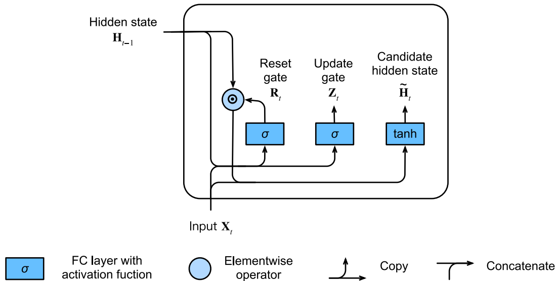
图9.1.2: 在门控循环单元模型中计算候选隐藏状态。
