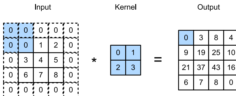
图6.3.1: 带填充的二维互相关。
