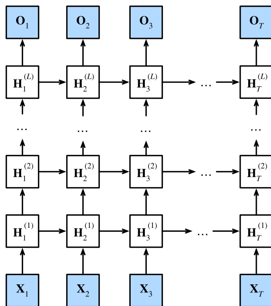
图9.3.1: 深度循环神经网络的结构。
