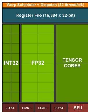
图10.4.7: NVIDIA Turing 处理块（图片由英伟达提供）
