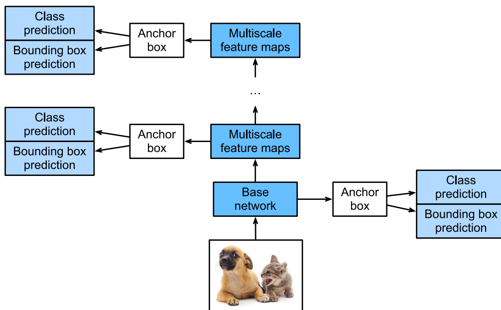
图11.7.1: 单发多框检测模型主要由一个基础网络块和若干多尺度特征块串联而成。
