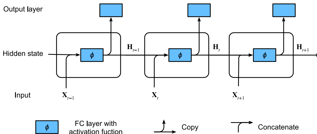
图8.4.1: 具有隐藏状态的循环神经网络。
