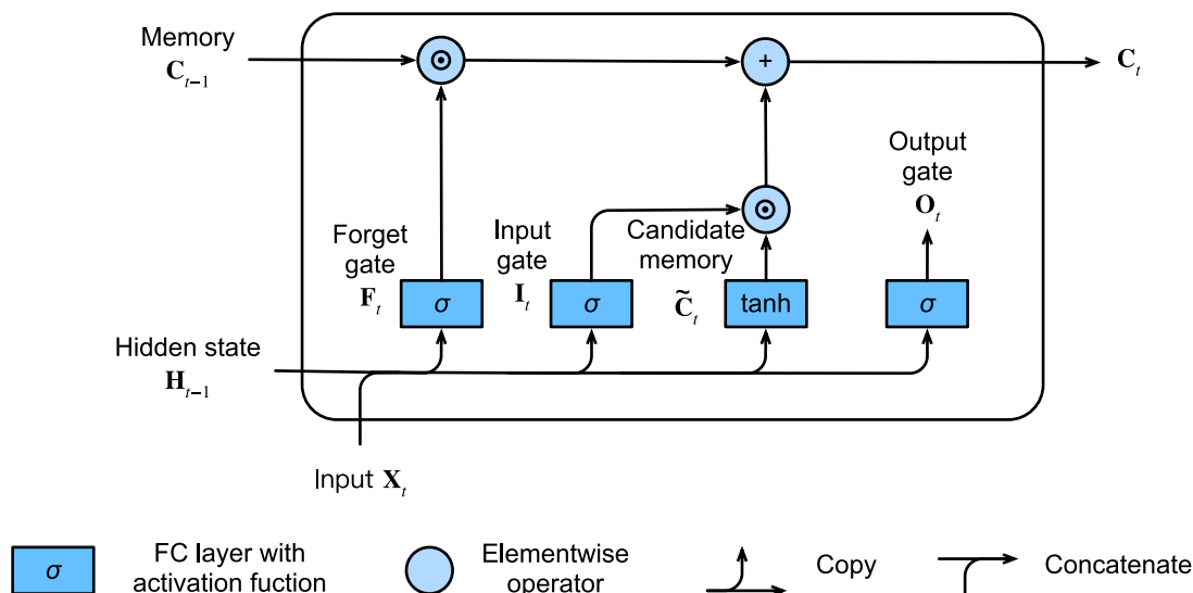
图9.2.3: 在长短期记忆网络模型中计算存储单元。
