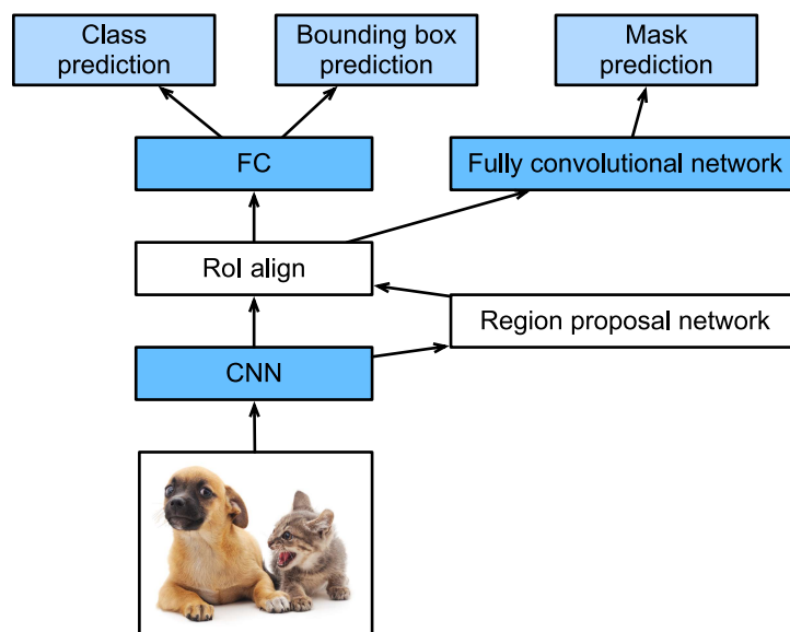
图11.8.5: Mask R-CNN 模型
