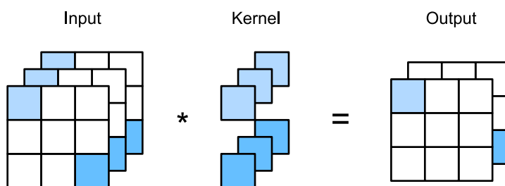
图6.4.2: 互相关计算使用了具有3个输入通道和2个输出通道的 1 \times 1 卷积核。其中，输入和输出具有相同的高度和宽度。
