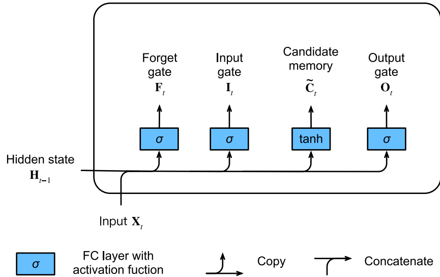
图9.2.2: 在长短期记忆模型中计算候选记忆单元。
