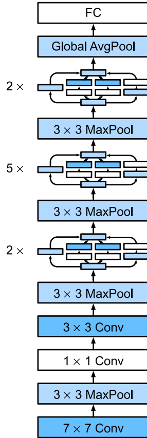
图7.4.2: GoogLeNet结构。
