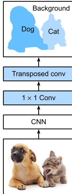
图11.11.1: 全卷积网络
