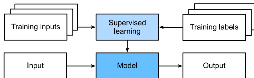
图1.3.1: 监督学习
