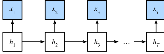
图9.4.1: 隐马尔可夫模型。
