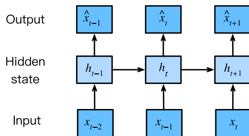
图8.1.2: 隐变量自回归模型
