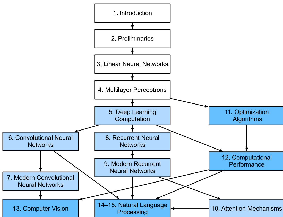
图1: 全书结构
