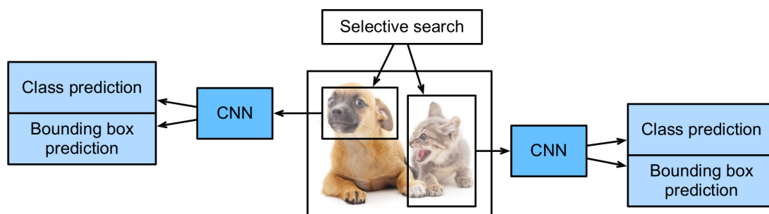
图11.8.1: R-CNN模型
