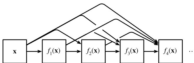
图7.7.2: 稠密连接。
