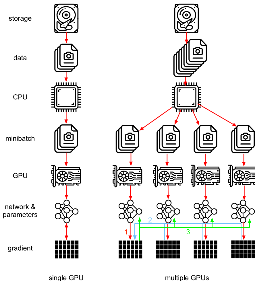
图10.7.1: 左图：单GPU训练。右图：多GPU训练的一个变体：（1）计算损失和梯度，（2）所有梯度聚合在一个GPU上，（3）发生参数更新，并将参数重新广播给所有GPU。
