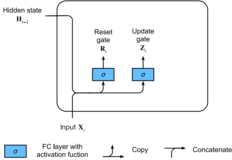
图9.1.1: 在门控循环单元模型中计算重置门和更新门。
