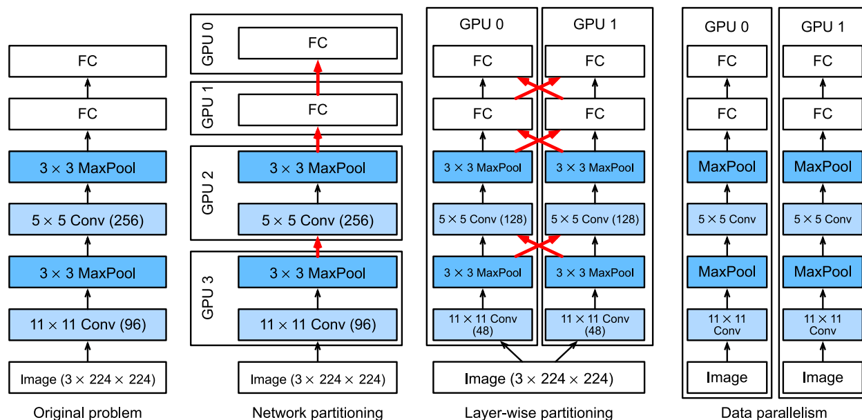
图10.5.2: 在多个GPU上并行化。从左到右：原始问题、网络并行、分层并行、数据并行。
