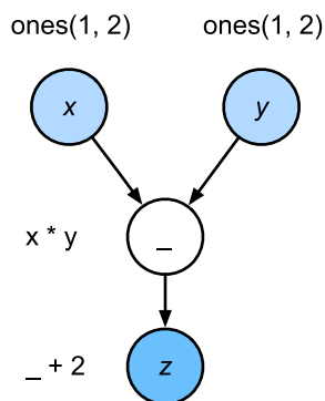
图10.2.2: 后端跟踪计算图中各个步骤之间的依赖关系。
