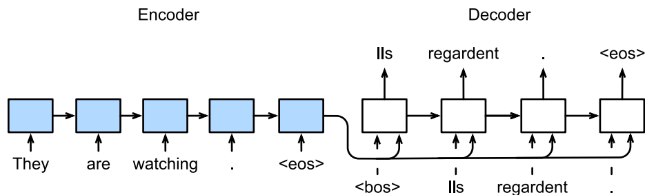
图9.7.1: 使用循环神经网络编码器和循环神经网络解码器的序列到序列学习。
