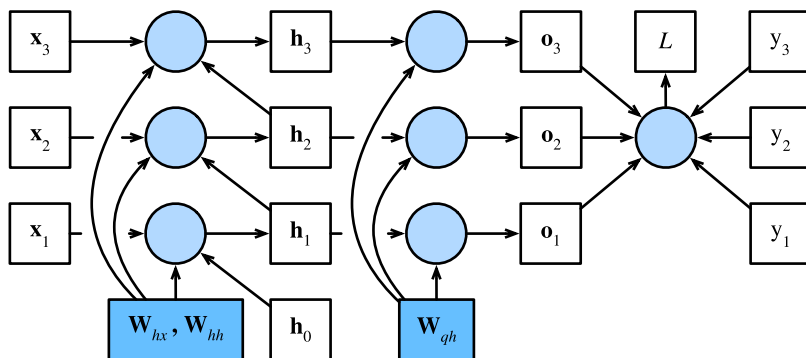
图8.7.2: 显示具有三个时间步的循环神经网络模型依赖关系的计算图。框表示变量（未着色）或参数（着色），圆表示运算符。
