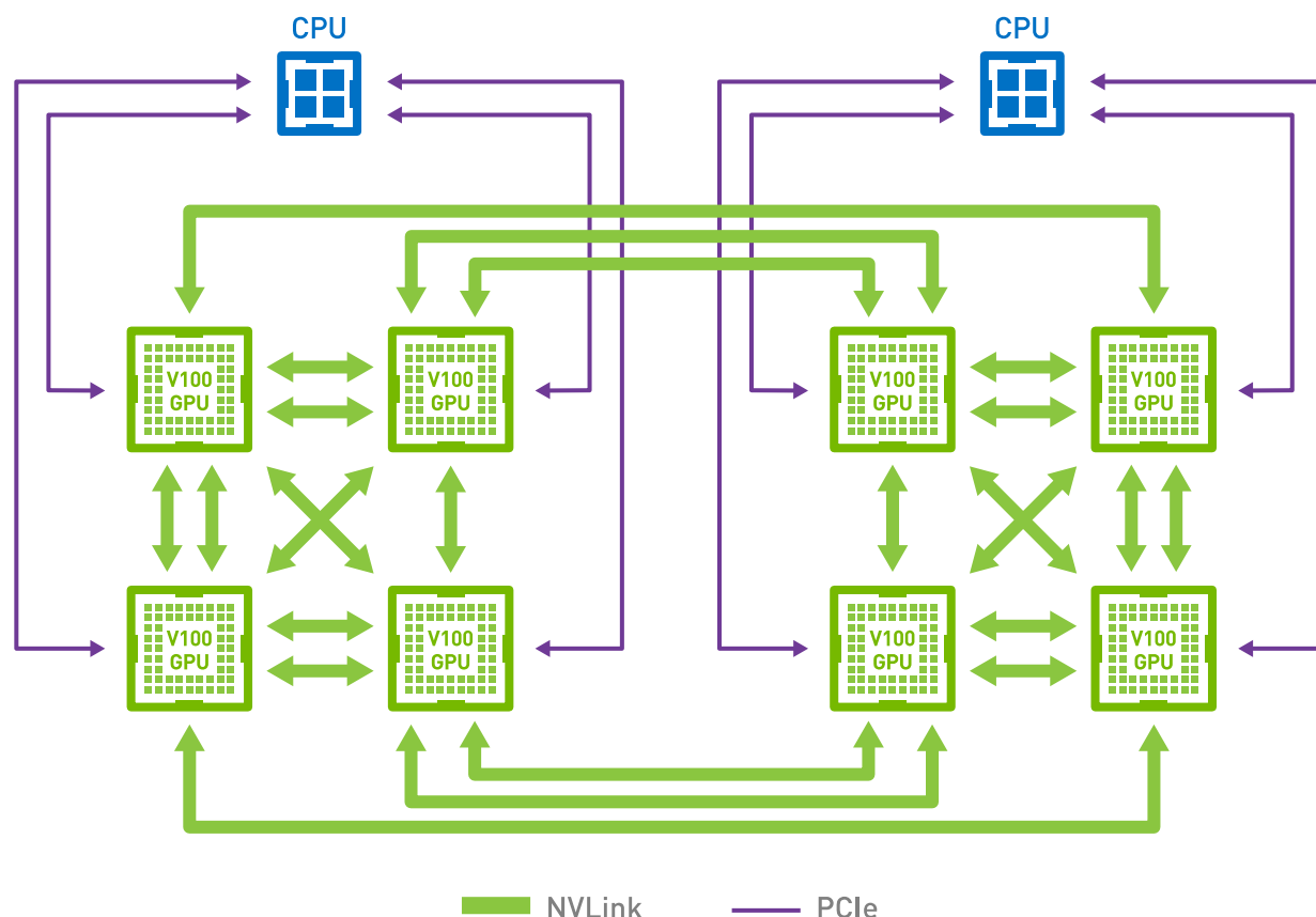
图10.7.4: 在 8 台 V100 GPU 服务器上连接 NVLink（图片由英伟达提供）
