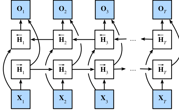
图9.4.2: 双向循环神经网络的结构。
