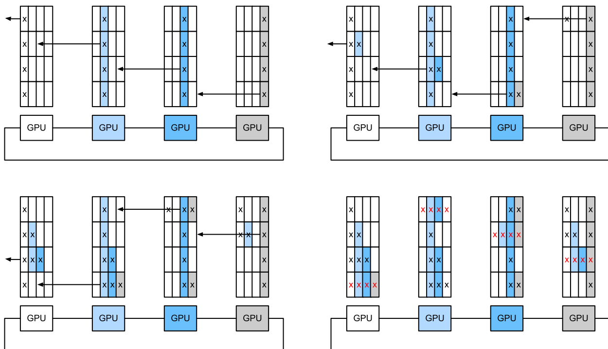
图10.7.6: 跨4个节点的环同步。每个节点开始向其左邻居发送部分梯度，直到在其右邻居中找到聚合的梯度。
