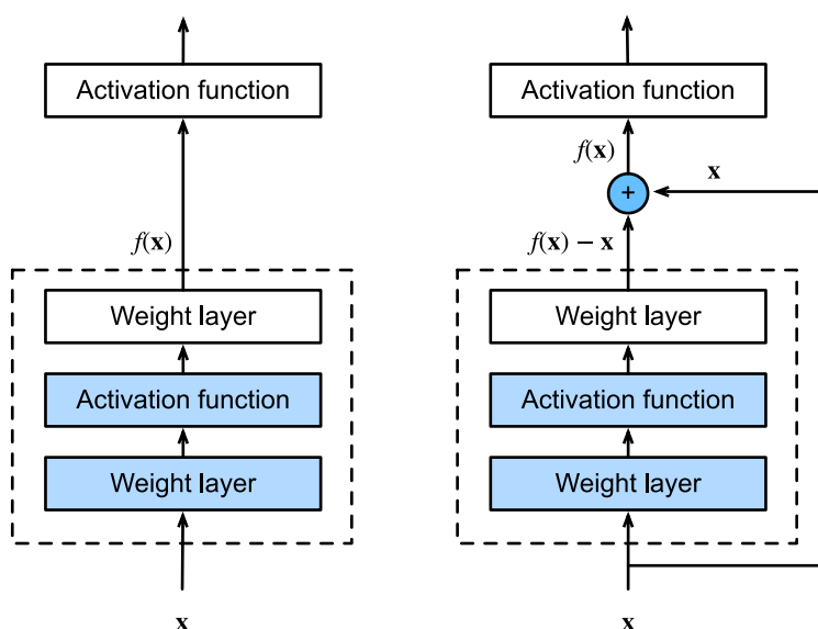
图7.6.2: 一个正常块（左图）和一个残差块（右图）。
