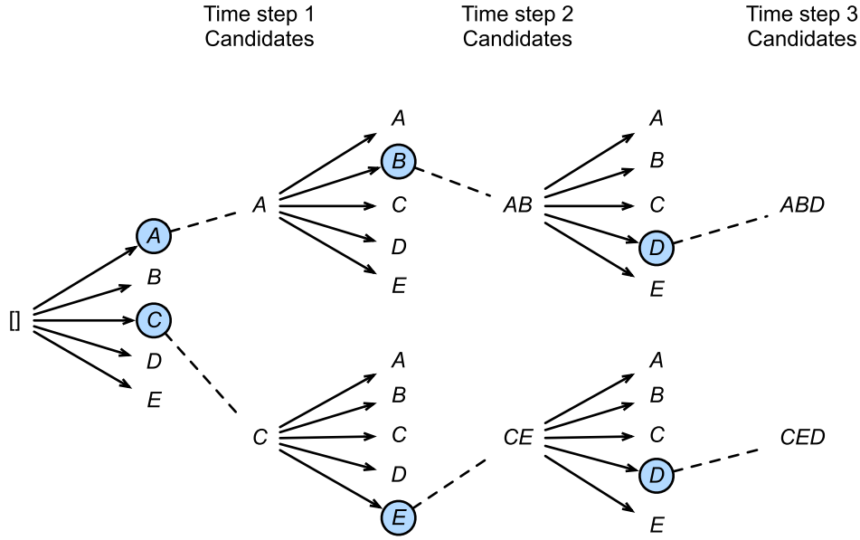
图9.8.3: 束搜索过程（束宽：2，输出序列的最大长度：3）。候选输出序列是A、C、AB、CE、ABD和CED。
