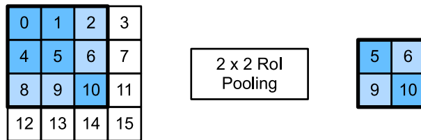
图11.8.3: 一个 2 \times 2 的兴趣区域池化层
