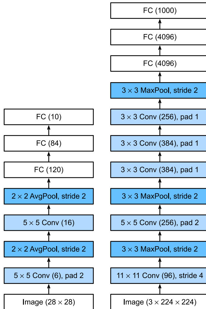
图7.1.2: 从LeNet（左）到AlexNet（right）
