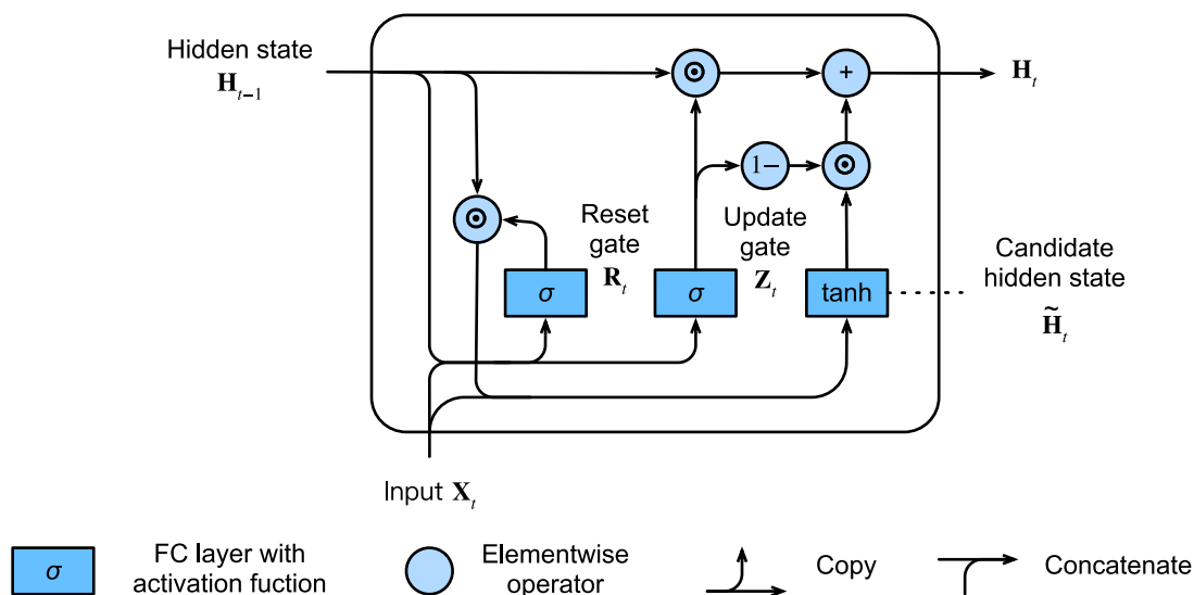
图9.1.3: 计算门控循环单元模型中的隐藏状态。
