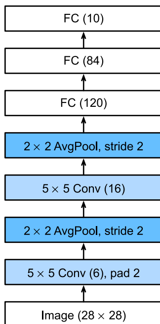
图6.6.2: LeNet 的简化版。
