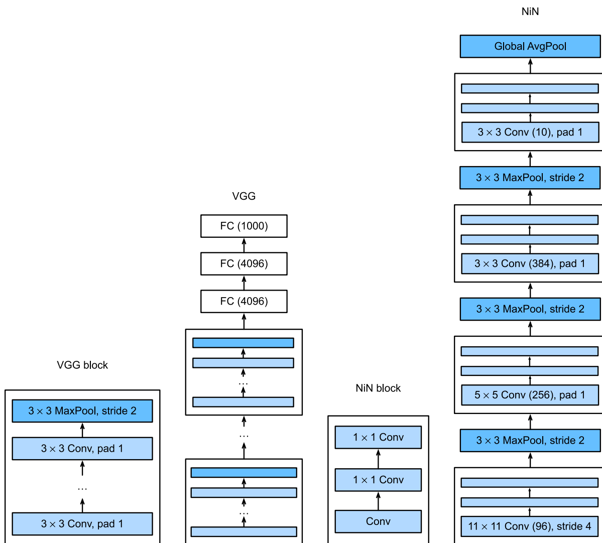
图7.3.1: 对比 VGG 和 NiN 及它们的块之间主要结构差异。
