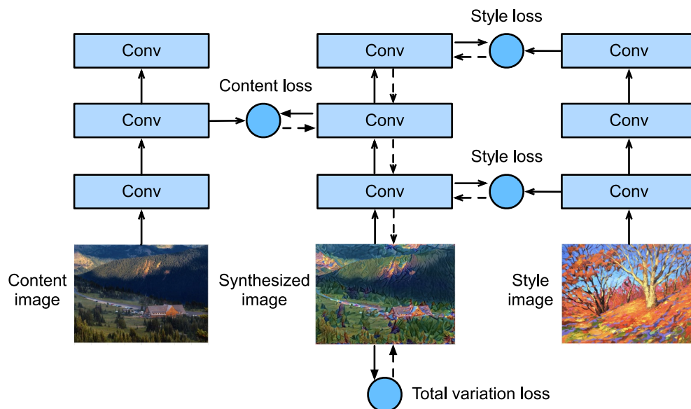
图11.12.2: 基于卷积神经网络的样式迁移。实线箭头和虚线箭头分别表示正向传播和反向传播
