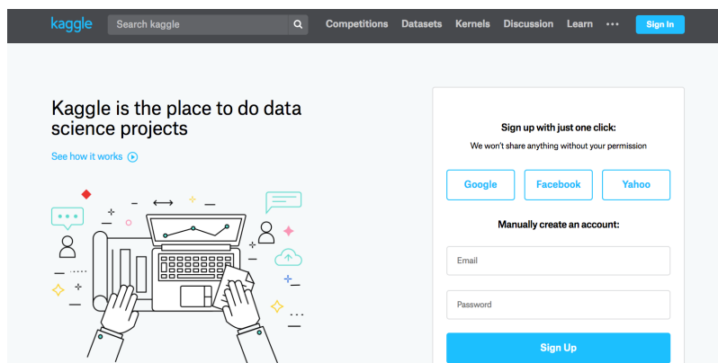
图4.10.1: Kaggle网站
