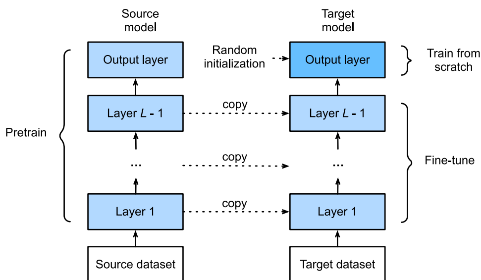
图11.2.1: 微调。
