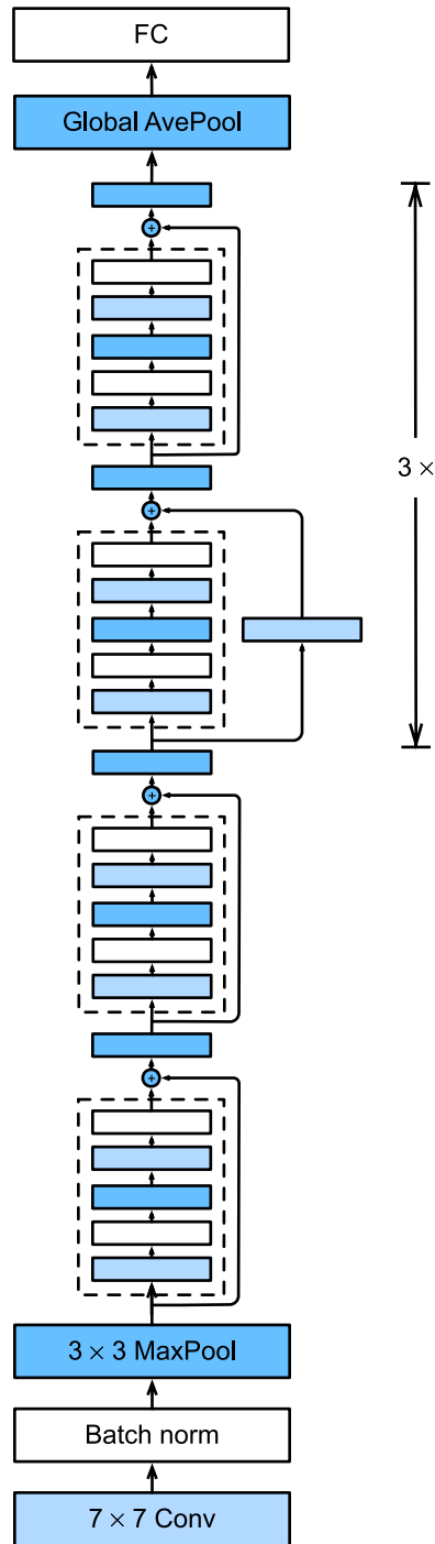
图7.6.4: ResNet-18 架构
