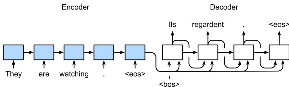
图9.7.3: 使用循环神经网络编码器-解码器逐标记地预测输出序列。
