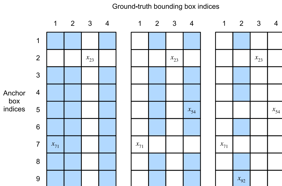
图11.4.2: 将真实边界框分配给锚框。
